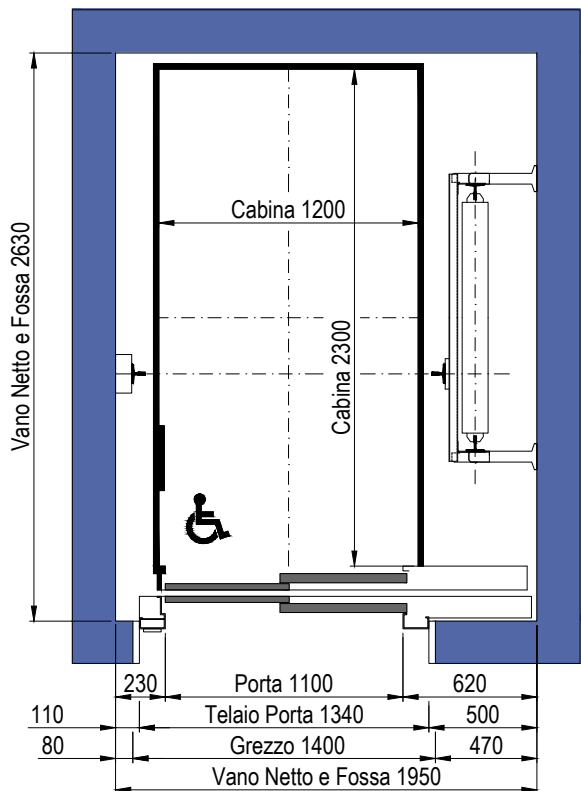
PIANTA VANO CORSA TELAIO PORTE DA 120mm
