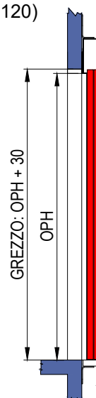
SEZIONE PORTA SENZA TELAIO (EI120)
